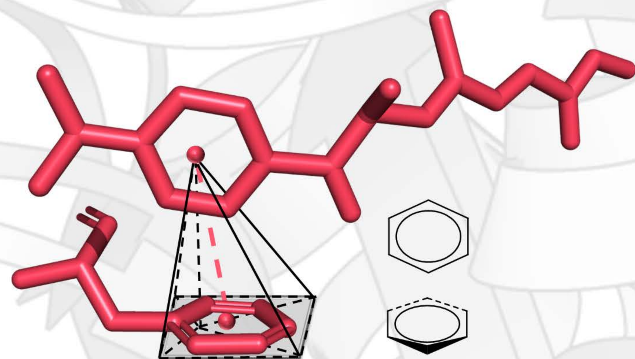
F202 (HDAC6)
